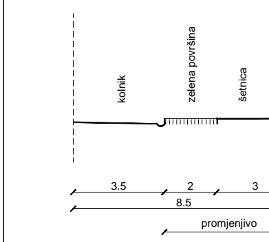
KARAKTERISTIČAN POPREČNI PRESJEK C - C, MJ. 1:200
