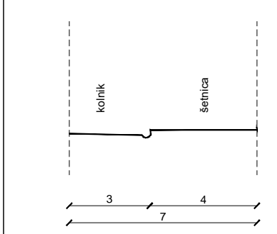
KARAKTERISTIČAN POPREČNI PRESJEK C - C, MJ. 1:200
