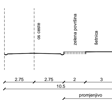
KARAKTERISTIČAN POPREČNI PRESJEK B - B, MJ. 1:200
